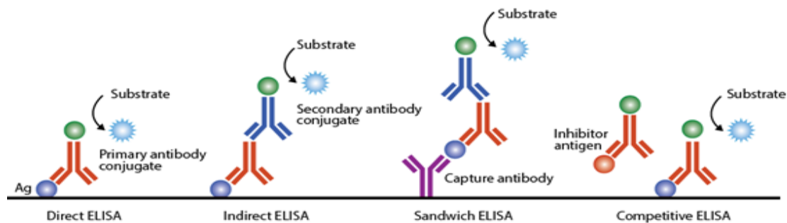
Slika 2.5.1. ELISA test
