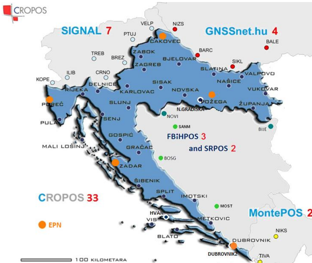
Slika 4.3. Položaj CROPOS referentnih stanica
