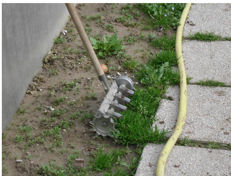
Slika 3.1.5. Četveroredna ručna sijačica kojom je obavljena sjetva rotkvice Foto: Mate Andrijašević
