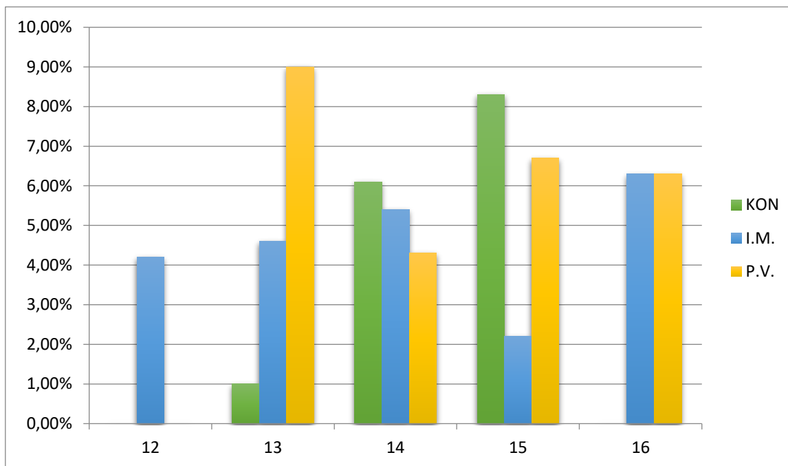
Grafikon 2. Udio avitalne prasadi (%) kod različitih načina indukcije prasenja s obzirom na veličinu legla
