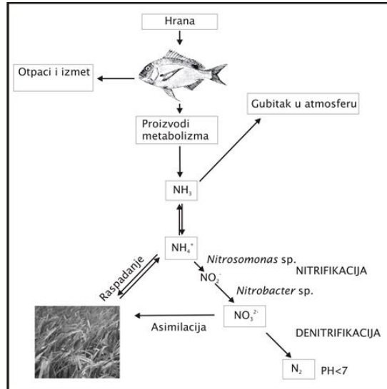
Slika 2: Dušični spojevi kao posljedica unosa organske tvari u procesu intenzivnog uzgoja ribe i procesi kruženja dušika u ekosustavu mora
