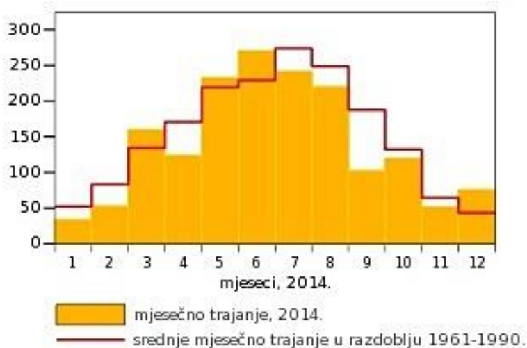
Slika 6: Insolacija (h), Zagreb-Maksimir
