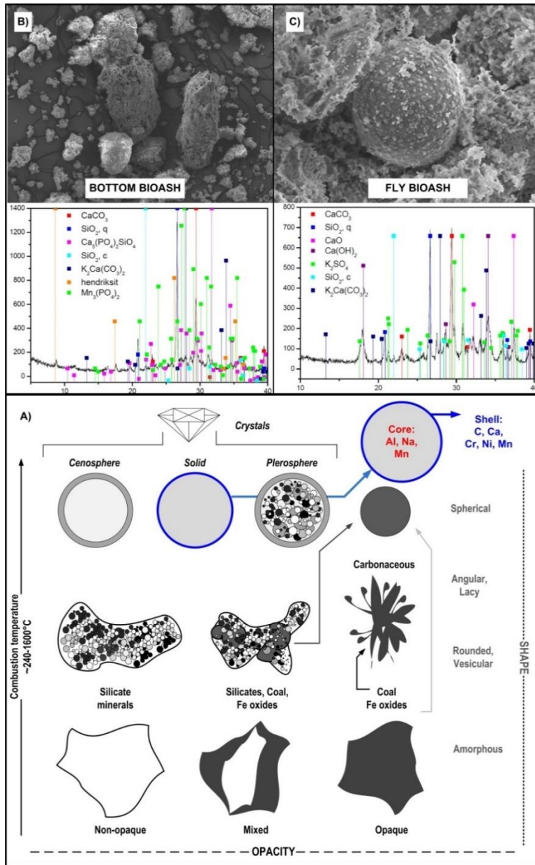
Slika 4.1. Snimke čestica biopepela sa dna ložišta i lebdećeg biopepela provedene skenirajućim elektronskim mikroskopom (SEM) i shematski prikaz njihovih glavnih morfoloških oblika.
