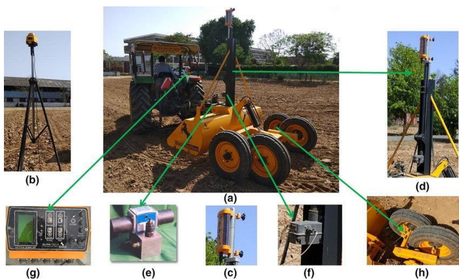
Slika 25. Dijelovi sustava laserskog navođenja: a) Laserski navođen priključni grejder b) Laserski odašiljač c) Laserski prijemnik d) Energetske jarbol e) Dvoradni magnetni prekidač f) Istosmjerni motor g) Senzor blizine smješten na h) kotačima (Ćosić, 2021).
