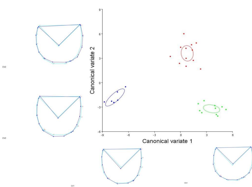
Slika 7. Prikaz vizualizacije rezultata CVA analize na grafu (crveno KL, zeleno ML, plavo ST) i razlike u obliku ljustaka sunčanice pomoću deformacijskih rešetki (CV1 i CV2, ekstremi 6 i -6)
