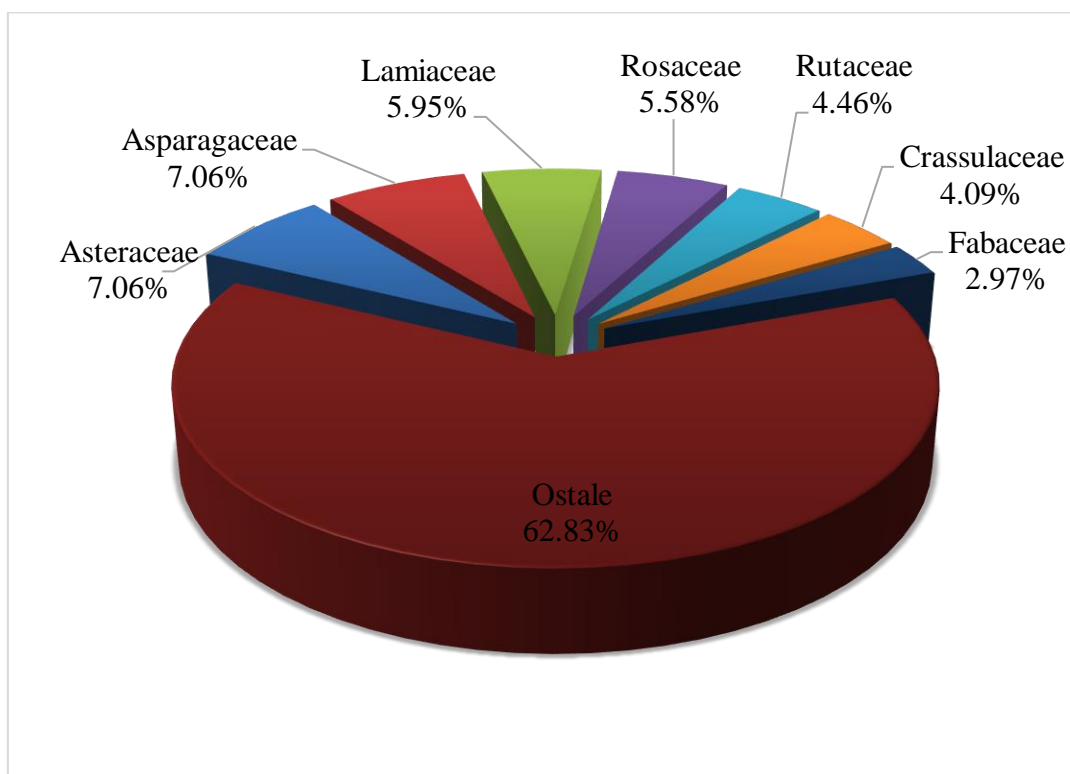
Grafikon 5.1. Zastupljenost porodica u vaskularnoj flori privatnih okućnica otoka Brača
