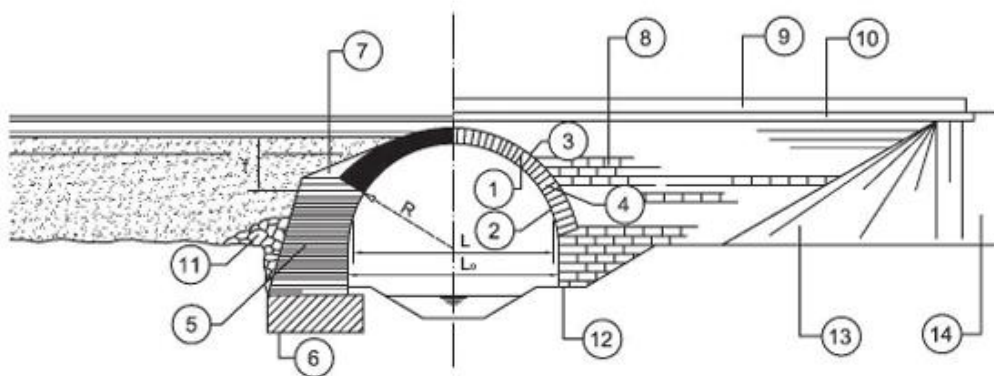
Slika 2.20. Poprečni presjek svođenog propusta (elementi: 1 – svod; 2 – intrados; 3 – ekstrados; 4 – peta svoda; 5 – upornjak; 6 – temelj; 7 – nazidak; 8 – čeonni zid; 9 – ograda; 10 – vijenac; 11 – kameni nabačaj; 12 – profil kanala; 13 – čunj; 14 – prilaz mostu; L – raspon svoda; L_0 – otvor propusta; r – radijus zakrivljenosti svoda; f – strelica svoda) (Izvor: Cerić i sur., 2022.)
