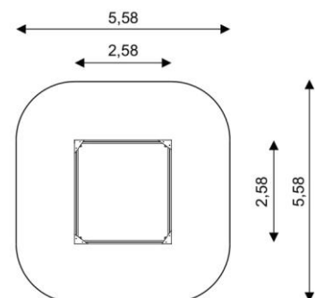
Slika 8.28. Tlocrt sprave
