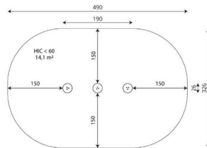
Slika 8.26. Tlocrt sprave
