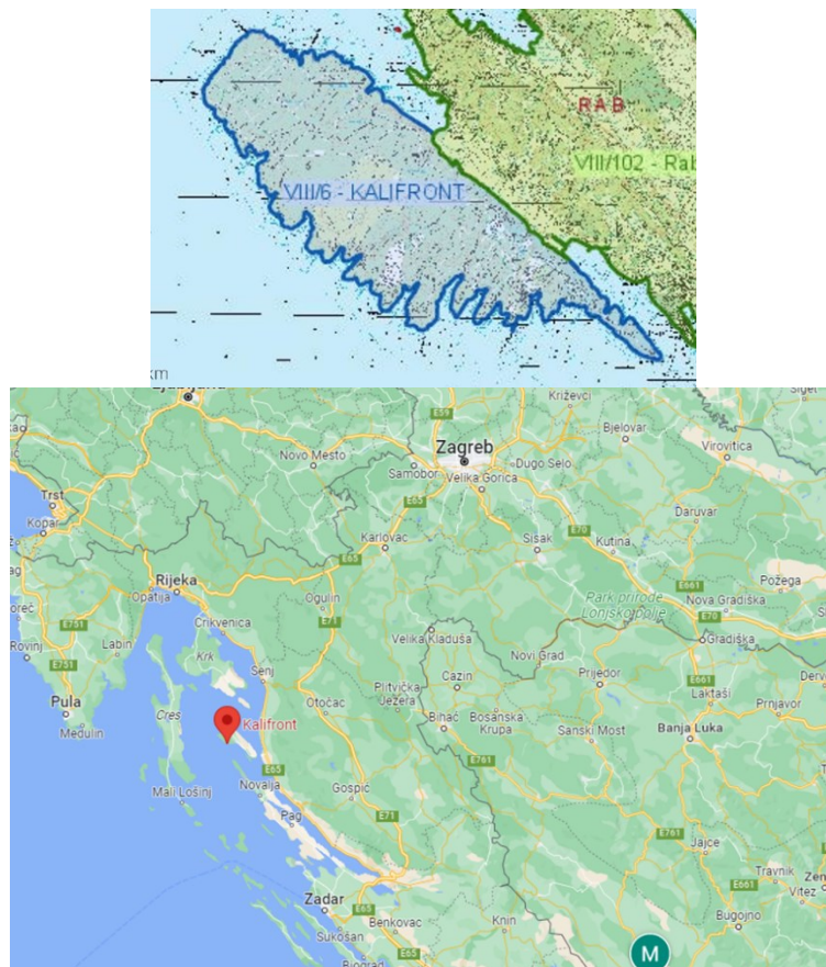
Slika 3.1.1. Karta s lokacijom otvorenog državnog lovišta Kalifront
