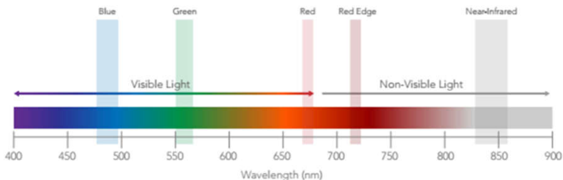
Slika 12. Spektralno područje senzora Micasense RedEdge.MXTM (Izvor: https://micasense.com/rededge-mx/ )
