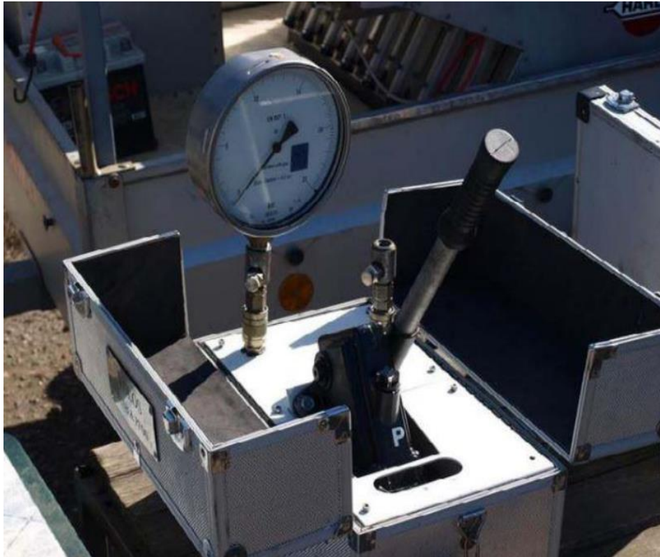
Slika 9. Uređaj za mjerenje ispravnosti rada manometra (Izvor: www.savjetodavna.hr )
