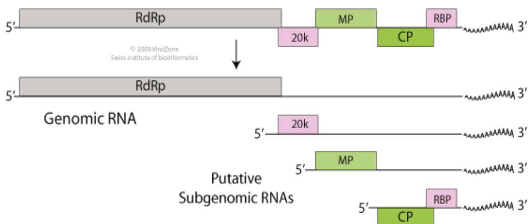
Slika 2.2.1.1. Organizacija genoma vitivirusa. Oznake: RdRp – enzim replikaza (replicase); 20k – nekodirajuća regija veličine 20000 parova baza; MP – protein za kretanju (movement protein); CP – protein omotača (coat protein)
