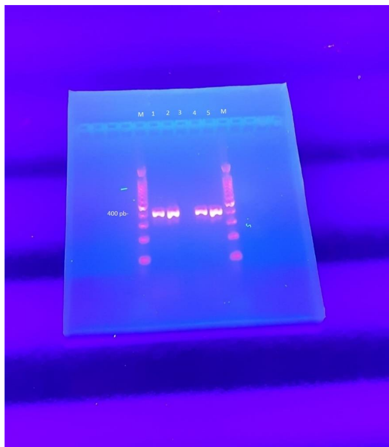
Slika 4.2. Rezultati testiranja metodom konvencionalnog RT-PCR-a na prisutnost GVH. Amplikoni 1 i 2 dobiveni su korištenjem CP početnica, dok su amplikoni 3 i 4 dobiveni korištenjem početnica za RdRp regiju. Prikazani amplikoni odgovaraju očekivanoj veličini PCR-produkta od 400 parova baza
