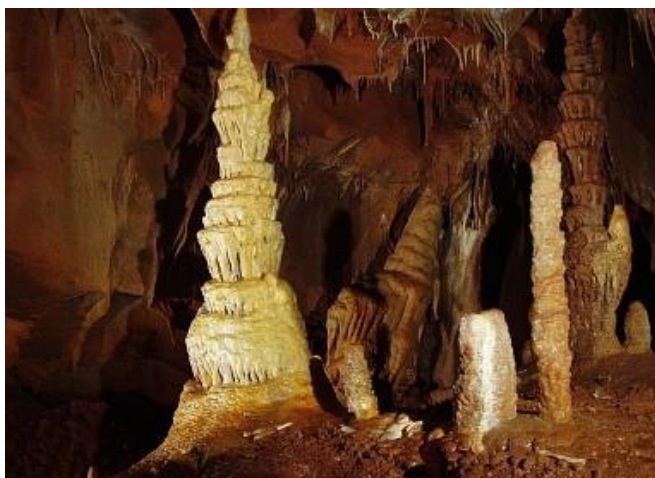
Slika 4.2.2.: Stalagmiti
