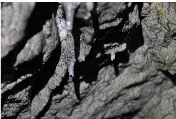
Slika 6.2.1.9.: Stalaktiti
