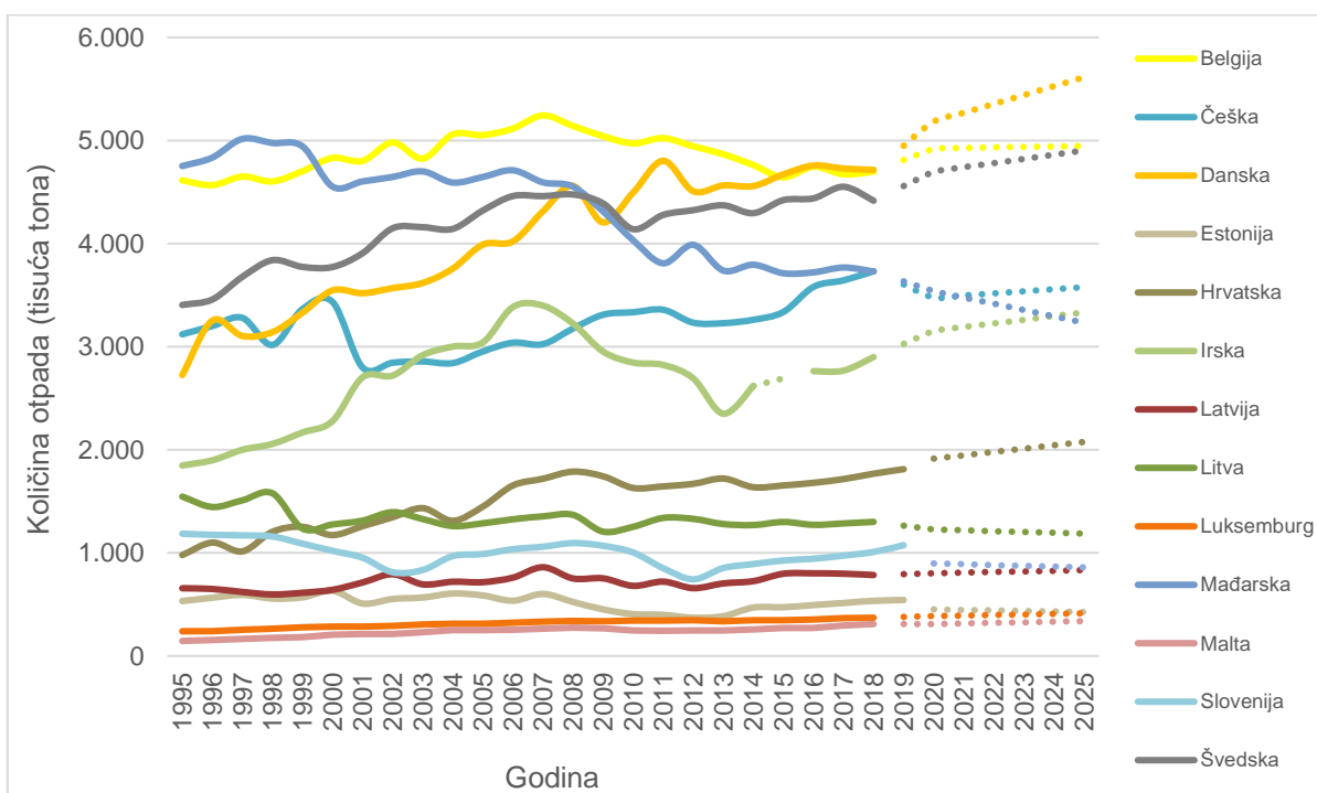
Slika 35. Količine nastaloga komunalnog otpada, prikaz u tisućama tona, za preostalih 13 promatranih država EU-a od 1995. do 2025. godine. Podaci označeni točkastim nizom predstavljaju vrijednosti dobivene ANN modelom.
