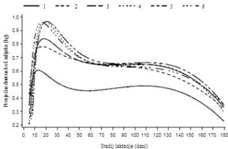
Slika 2.4.1. Laktacijska krivulja Ali-Schaeffer dnevni količina mlijeka paške ovce ugnježdene unutar redoslijeda laktacije
