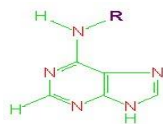
Slika 3.3. Struktura citokinina
