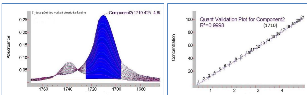
Grafikon 5. Referentna apsorpcijska vrpca / apsorbanacija na 1710\text{ cm}^{-1} (lijevo) koja pokazuje najbolje rezultate korelacije između stvarnog udjela stearinske kiseline u smjesama i instrumentalne predikcije udjela stearinske kiseline (desno: quant validation plot - brojevi od 1 do 21 odnose se na smjese s udjelom stearinske kiseline od 0 do 100 %)
