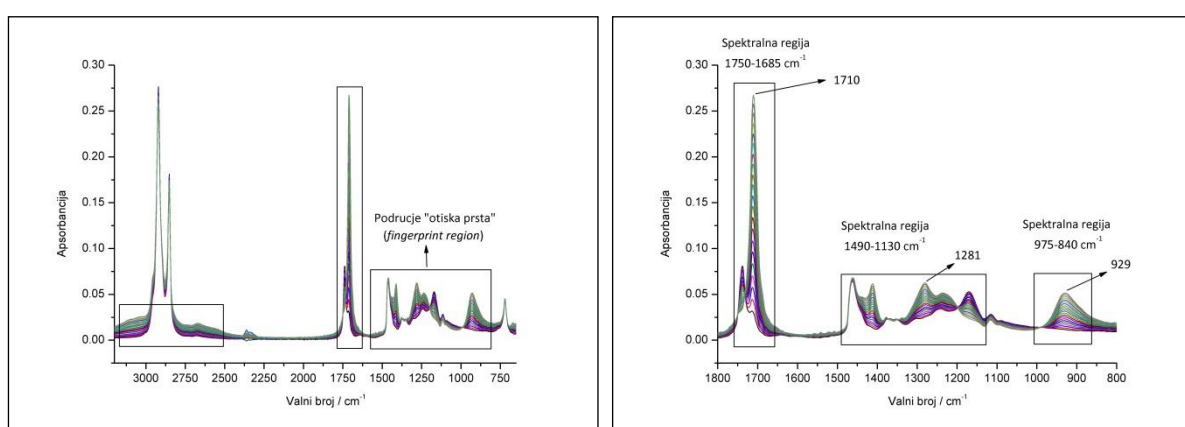
Grafikon 3. FTIR-ATR spektri smjesa pčelinjeg voska i stearinske kiseline s različitim udjelom stearinske kiseline (0 – 100 %): cijelo spektralno područje 3200\text{--}700\text{ cm}^{-1} (lijevo); fingerprint područje 1800\text{--}800\text{ cm}^{-1} (desno)
