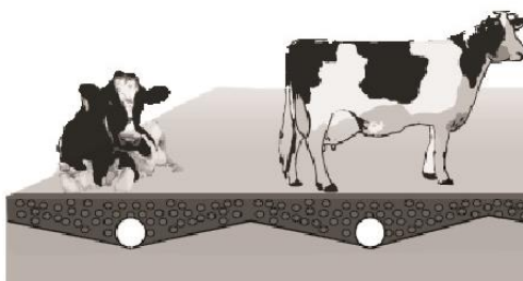
Slika 7.1.4.2. Prikaz propusne podnog madraca prema slojevima koji omogućuju odvajanje propuštanje tekućeg gnojiva, Izvor: Koentuin brošura, 2015., https://edepot.wur.nl/7959
