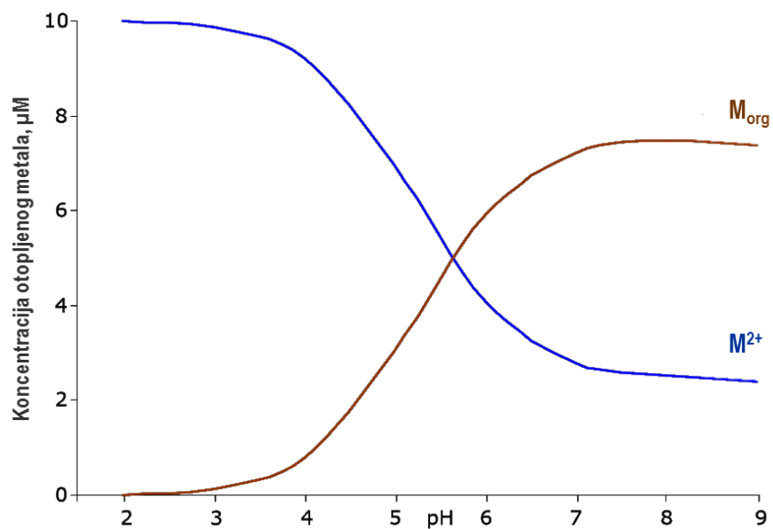
Slika 2. Shematski prikaz ovisnosti koncentracije većine slobodnih metalnih kationa ( M^{2+} ) u otopini tla i metala kompleksiranog s organskom tvari ( M_{org} ) o reakciji (pH) otopine tla pri povećanom udjelu organske tvari u tlu (prilagođeno prema Ondrašek, 2015).
