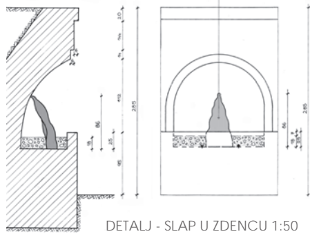
DETALJ - SLAP U ZDENCU 1:50
