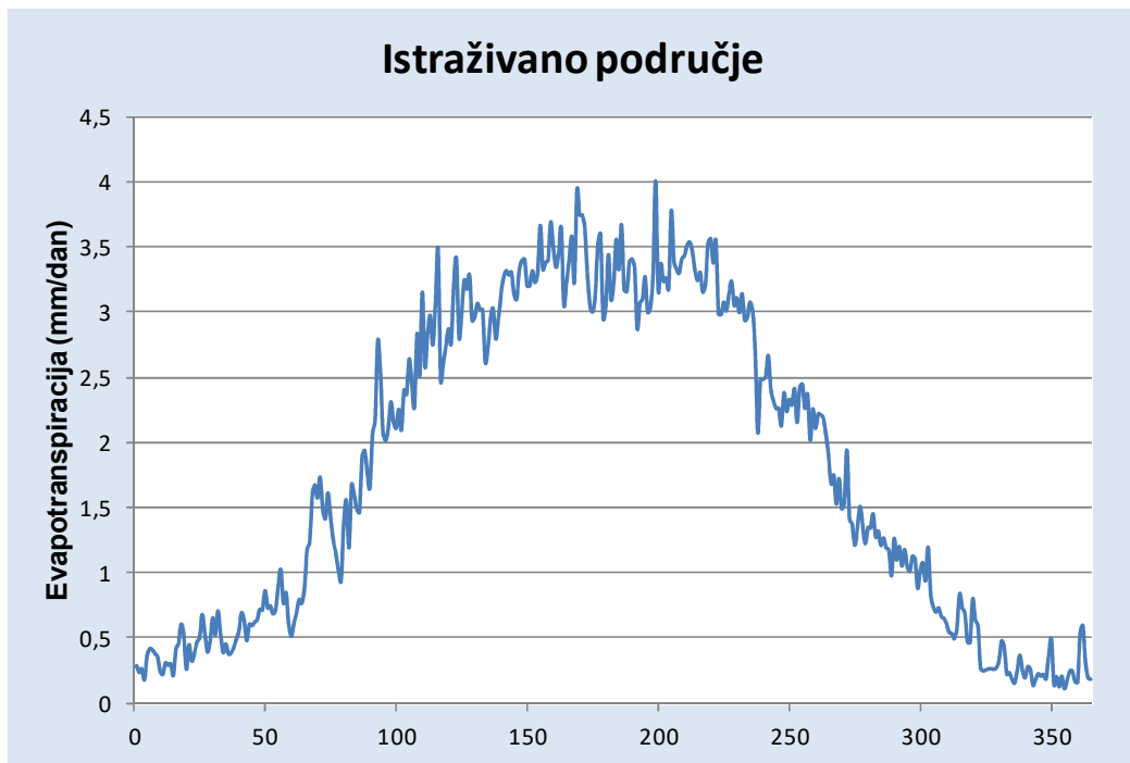
Slika 4.1.3. Prikaz evapotranspiracije na istraživanom području za 2018. godinu
