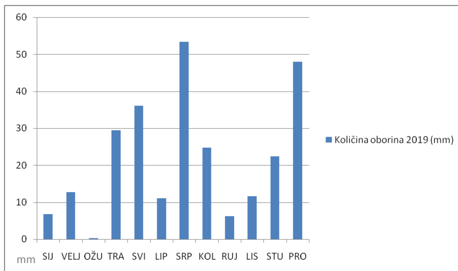
Graf 3.2.1.3. Prikaz količina oborina po mjesecima za 2019. godinu
