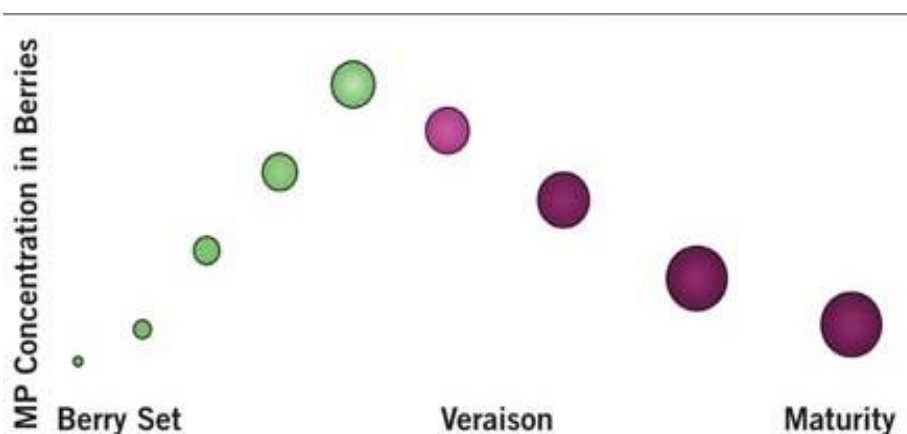
Slika 4. Koncentracija metokspirazina u bobi tijekom dozrijevanja
