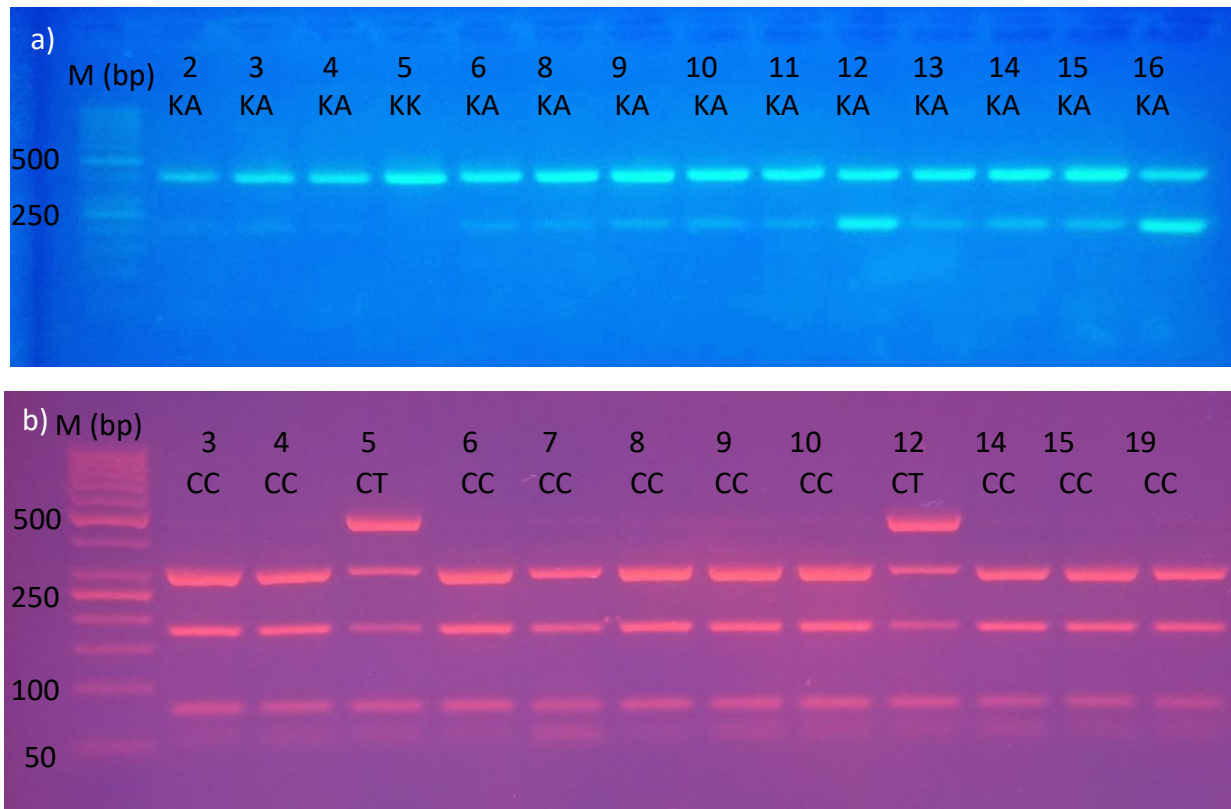
Slika 3.3. Dobiveni genotipovi: a) DGAT1 gena ( KA 411 bp, KK 208, 203 bp) i b) TG gena ( CC 295, 178, 75bp; CT 75, 178, 295, 473bp) križanaca belgijskog plavog i holštajn goveda. M – standard razmaka 100 bp; 2-16 i 3-19 – oznake uzoraka
