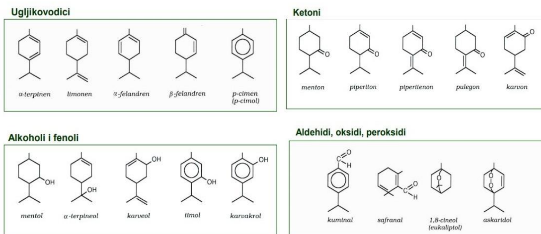
Slika 2.3. Monociklički monoterpeni
