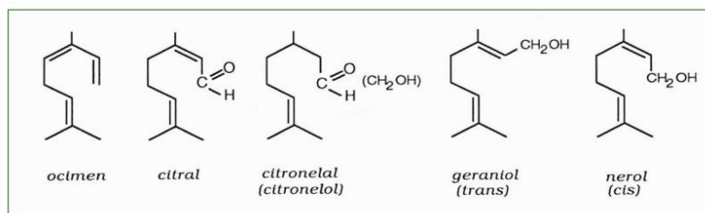
Slika 2.2. Aciklički monoterpeni
