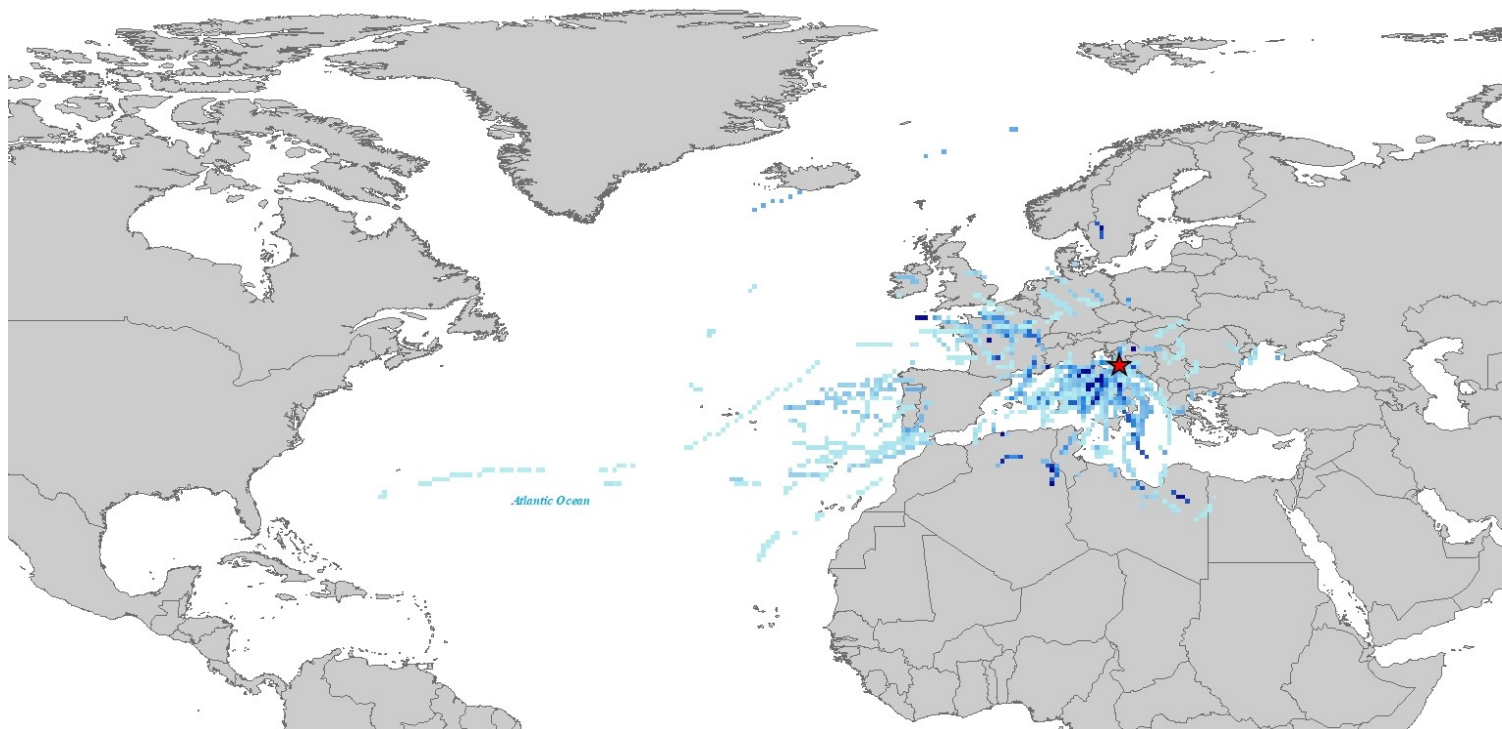
Slika 10: Lokacije izdizanja vlage duž 5-dnevnih unazadnih putanja zračnih masa za oborine iznad meteorološke postaje Zadar tijekom 2001. godine
