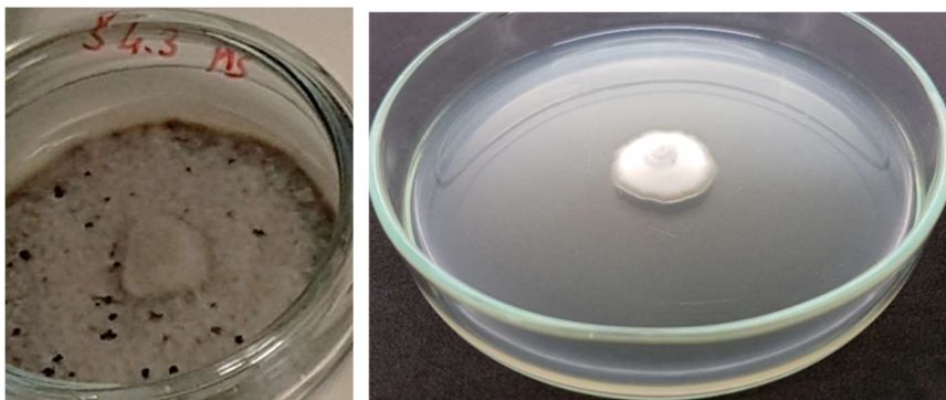
Slika 5.2.1. Izolati grupe 2: Š4.3 (lijevo) i Š7.4 (desno)
