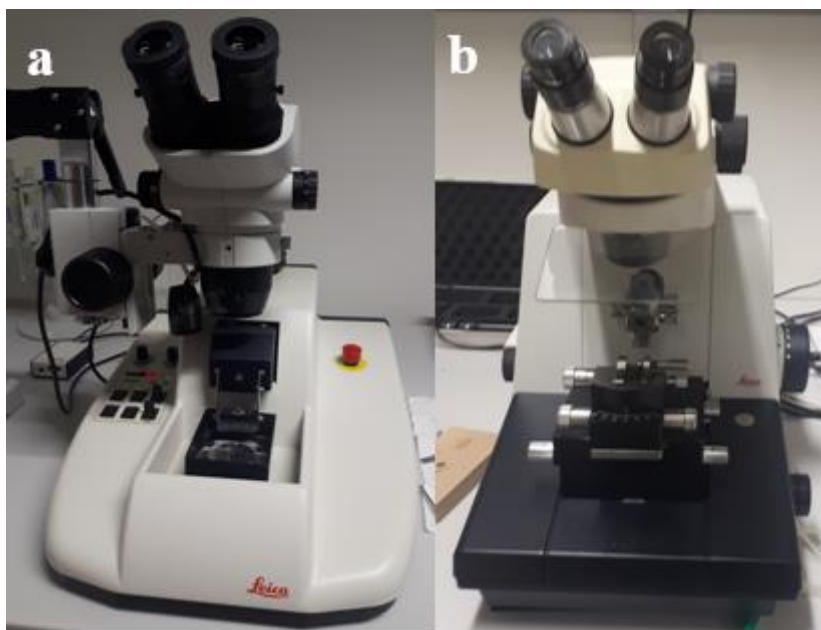
Slika 3.4.4.1. Uređaji za rezanje uzoraka: Vibratome (a) i Microtome (b)
