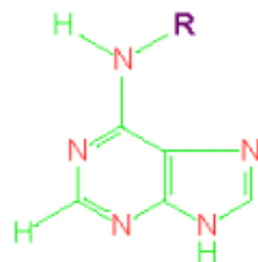
Slika 1.1. struktura citokinina
