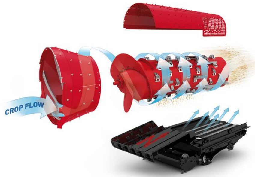
Slika 3.10. Aksijalni vršidbeni aparat sa jednim rotorom
