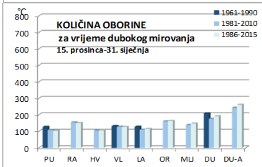
Slika 4.6. Količina oborine (mm) za vrijeme mirovanja masline, zime i dubokog mirovanja masline za odabrane postaje u razdobljima 1961. – 1990., 1981. – 2010. i 1986. – 2015. PU –Pula, RA – Rab, HV – Hvar, VL – Vela Luka, LA – Lastovo, OR – Orebić, MLJ – Mjet, DU – Dubrovnik i DU-A – Dubrovnik-aerodrom.
