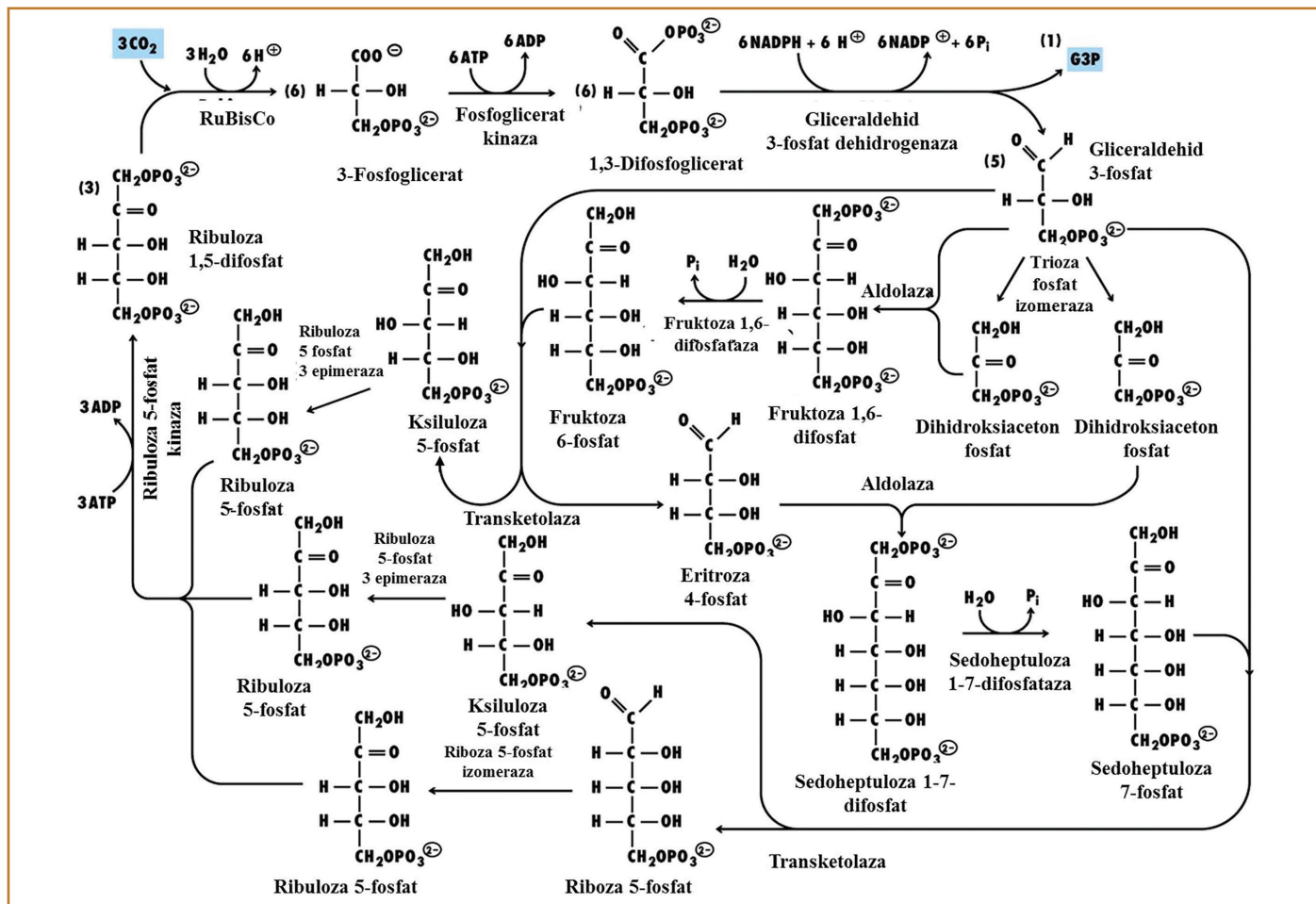
Slika 5.10. Reakcije Calvinova ciklusa.
