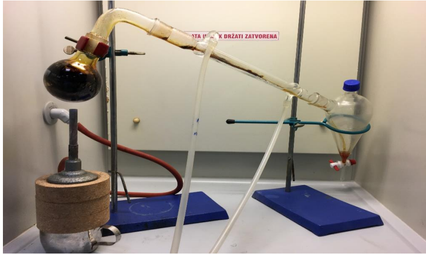
Slika 3.2.9.1. Piroliza
