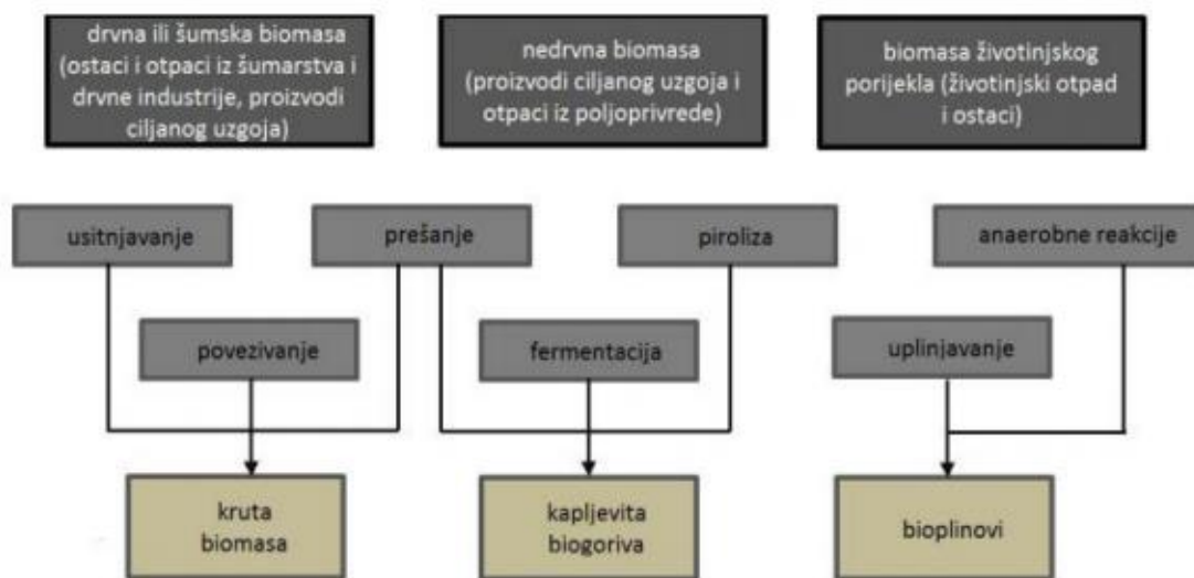
Slika 3.1. Proces dobivanja energije iz biomase Izvor: https://repozitorij.unin.hr/islandora/object/unin:1721/preview
