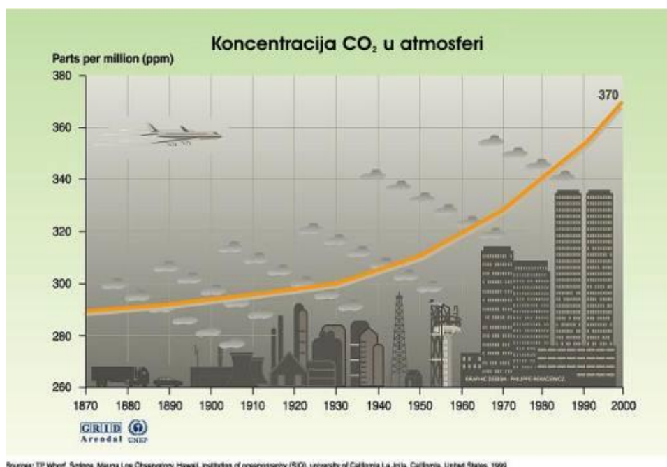
Slika 1.2. Porast koncentracije CO 2 u atmosferi kroz vremenski period u S.A.D.-u
