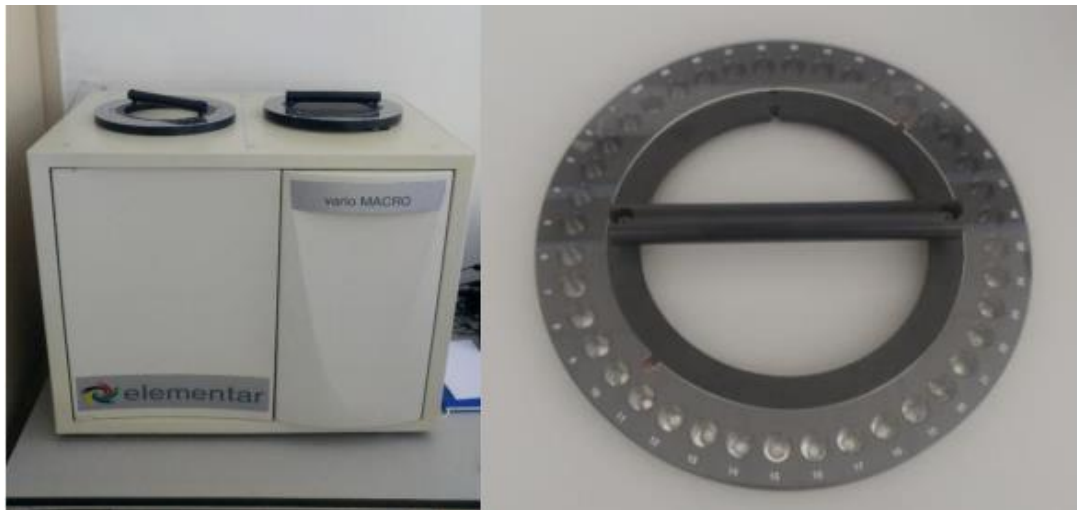
Slika 4.3. Prikaz CHNS analizatora s autosamplernom
