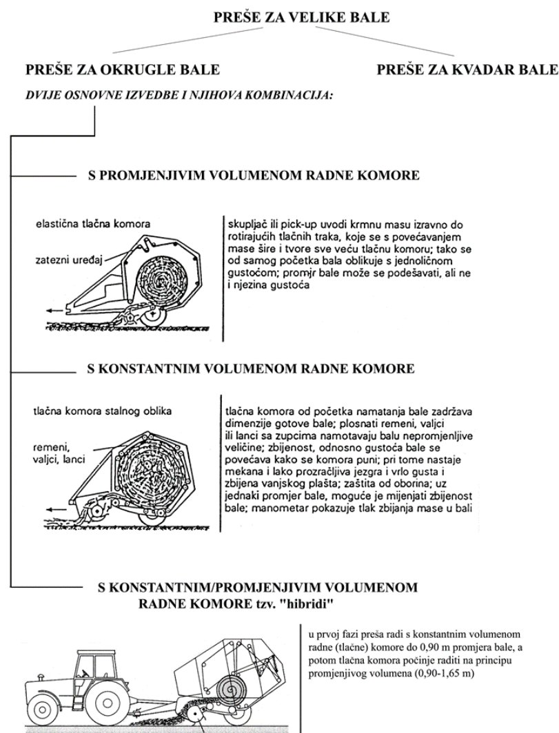
Slika 5. Preše za velike bale Izvor: Skripta Dubravko Filipović
