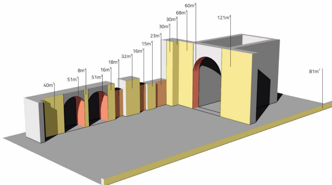
Slika br. 17 Strukturna analiza plohi osvjetljavanja
