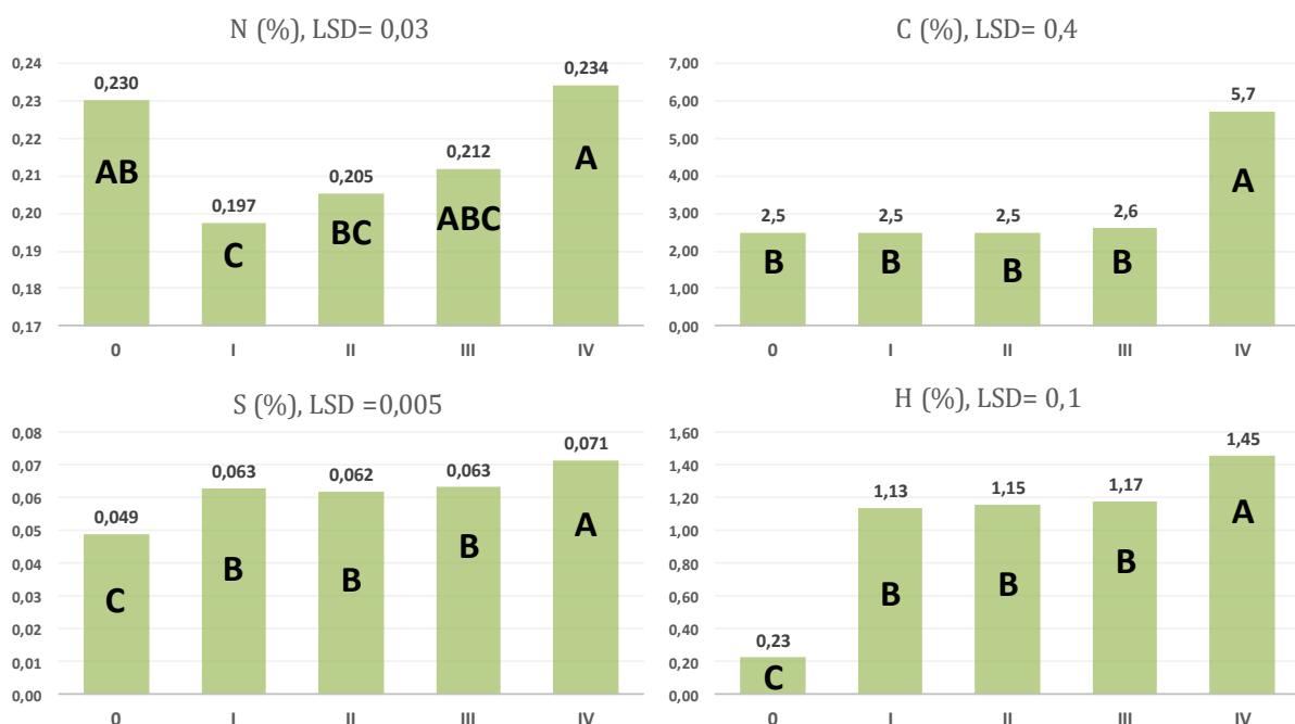
Slika 5.2.7. Rezultati statističke analize sadržaja N, C, S i H u tlu
