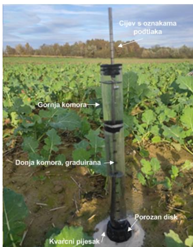
Slika 7. Prikaz mjerenja infiltracijske sposobnosti tla pomoću mini disk infiltrometra
