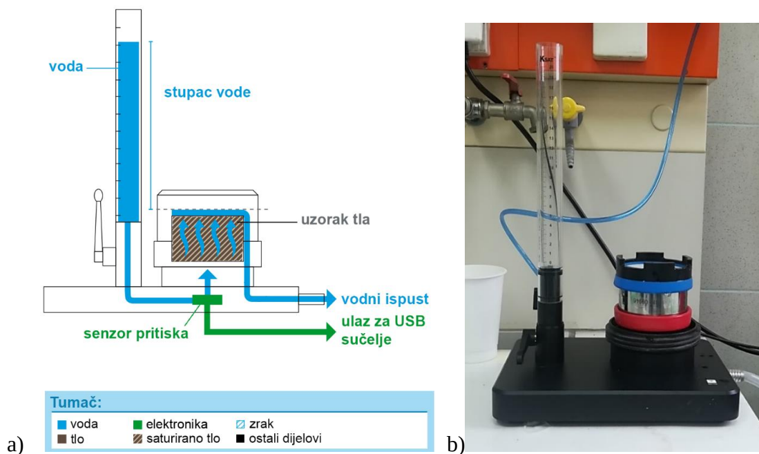
Slika 9. a) Shema K-SAT sustava i b) prikaz K-SAT sustava u MELILAB laboratoriju.
