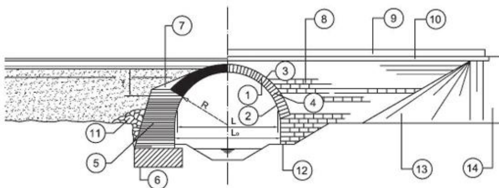
Slika 2.20. Poprečni presjek svođenog propusta (elementi: 1 – svod; 2 – intrados; 3 – ekstrados; 4 – peta svoda; 5 – upornjak; 6 – temelj; 7 – nazidak; 8 – čeoni zid; 9 – ograda; 10 – vijenac; 11 – kameni nabačaj; 12 – profil kanala; 13 – čunj; 14 – prilaz mostu; L – raspon svoda; L_0 – otvor propusta; r – radijus zakrivljenosti svoda; f – strelica svoda) (Izvor: Cerić i sur., 2022.)
