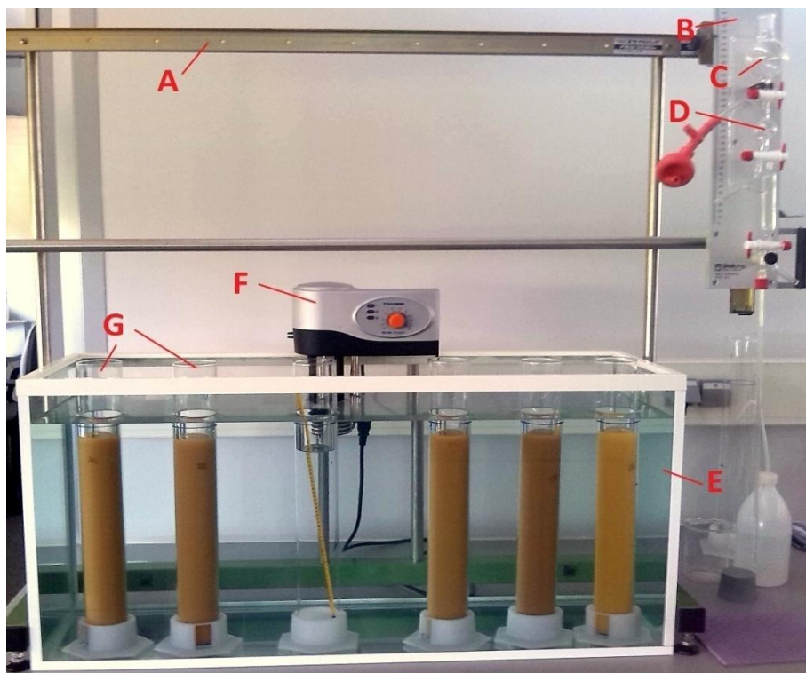
Slika 4: Pipet aparat za normiranu pipet metodu
