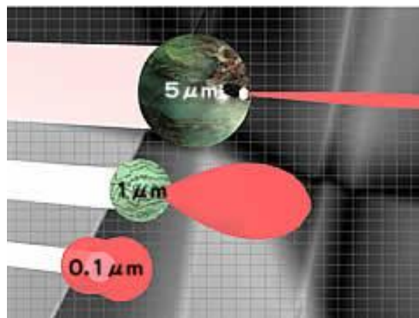
Slika 11: Intenzitet raspršenja laserske svjetlosti u ovisnosti od veličine čestica
