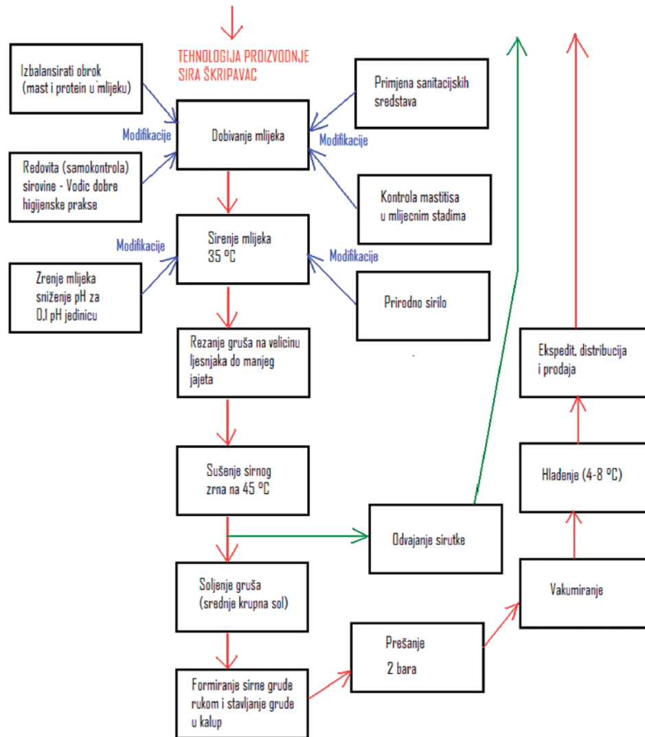
Slika 4. Shematski prikaz postupka proizvodnje sira škripavca
