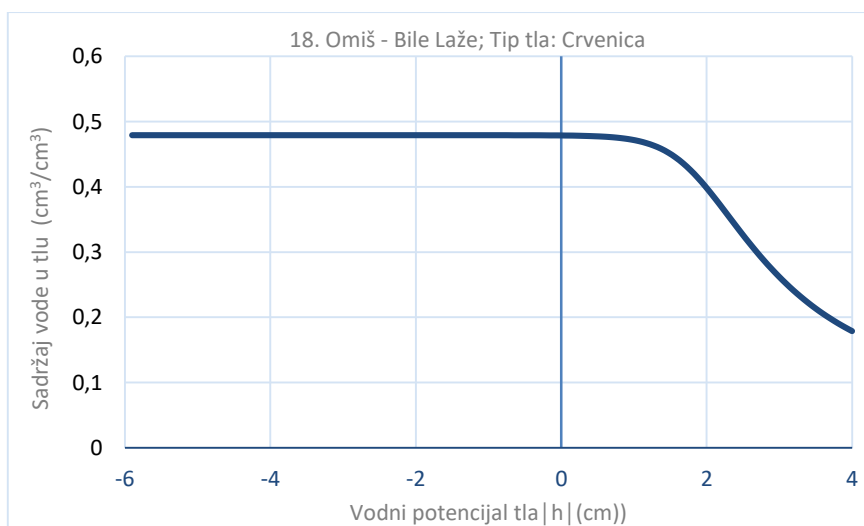
Slika 4.7. Retencijske krivulje količine vode u tlu (vlage u tlu) u programu HYDRUS na istraženim lokacijama u blizini Dubrovnika
