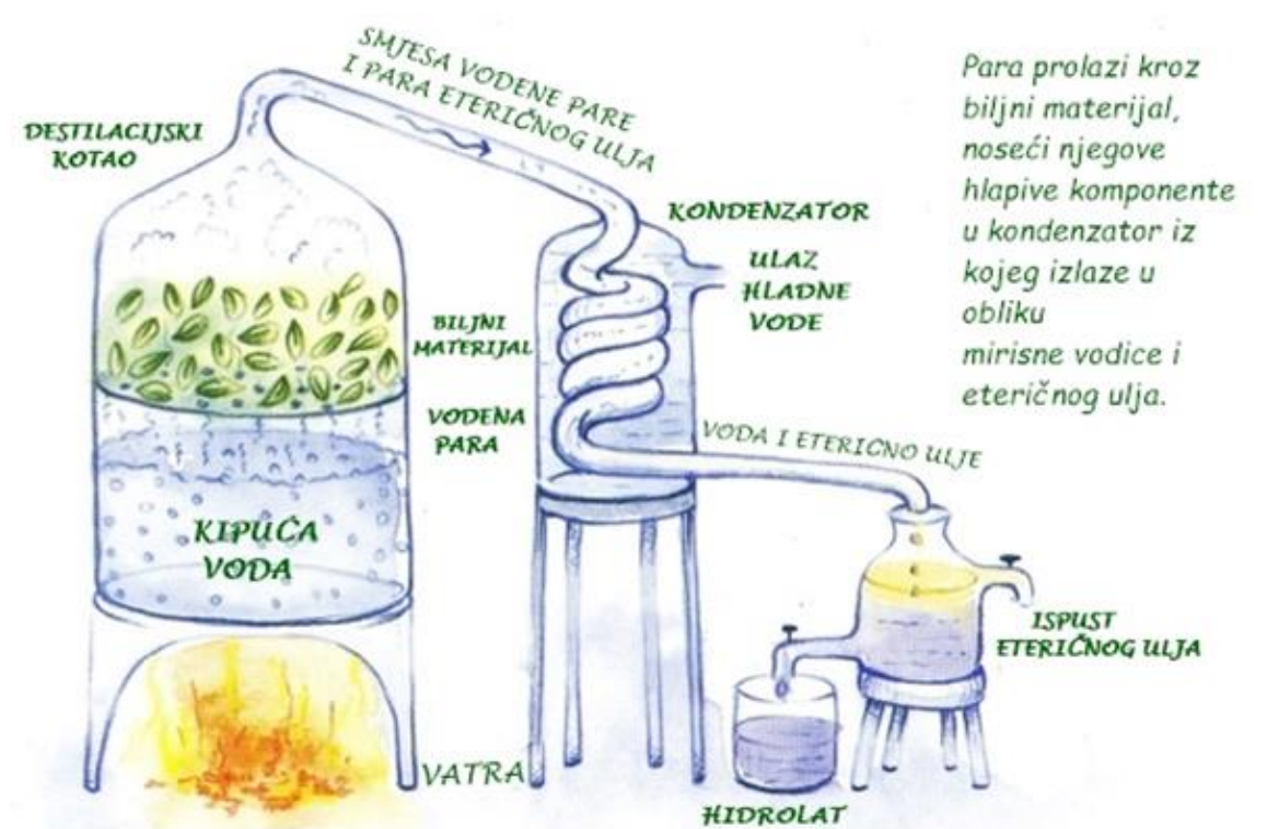
Slika 17. Prikaz destilacije vodenom parom (izvor originala: templesweep.com, 2015., autorska dorada)
