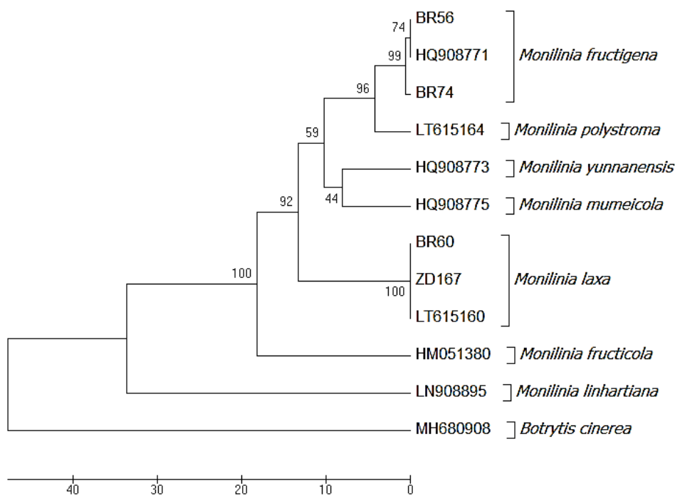
Slika 22. Filogenetsko stablo dobiveno analizom nukleotidnih sekvenci fragmenta gena za TUB2, uz korištenje UPGMA metode i modela ' number of differences '. Brojevi u čvorištu grana predstavljaju vrijednosti dobivene statističkom metodom ' bootstrap ' uz 1000 ponavljanja. Za ukorjenjivanje stabla korištena je sekvenca vrste B. cinerea , a u analizu su uvrštene i sekvence drugih Monilinia vrsta. Na stablu su vidljivi pristupni brojevi sekvenci iz baze podataka GenBank (Tablica 13) te oznake izolata iz ovog istraživanja (Prilog 4).
